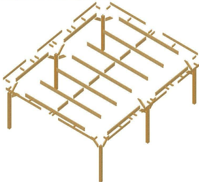
Représentation éclatée ossature toit plat standard en bois douglas FRANCE.
